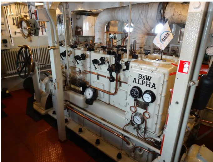
Hovedmaskinen i det meget velholdte maskinrum på "MØN"
